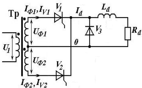
Рис. 1-4 Двухфазная нулевая схема выпрямления с шунтирующим диодом
