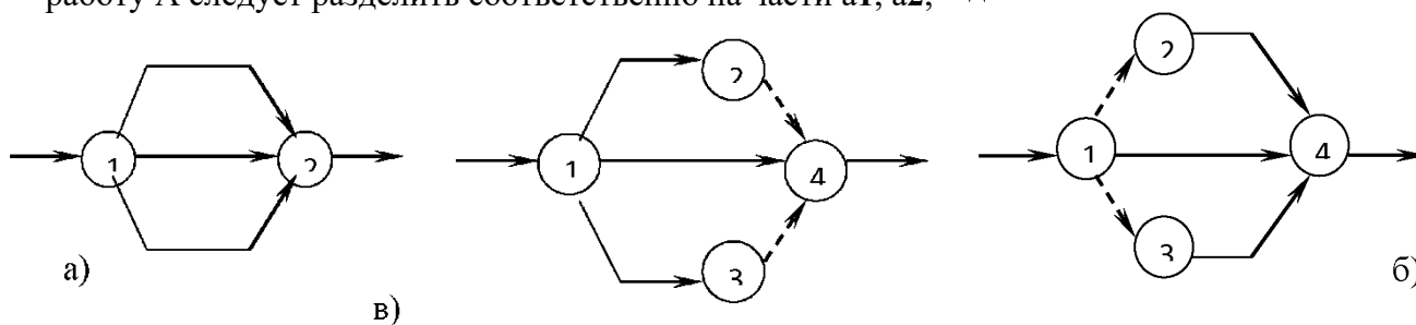
Рис. 1. Изображение параллельных работ в сети: а - неправильное; б - правильное. При этом каждая часть работы А считается самостоятельной работой и имеет свои предшествующие и последующие события (рис. 2). Таким приемом пользуются при изображении поточной организации труда на захватках.
