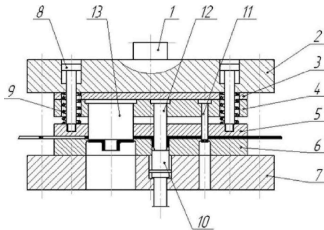
Рис. 7-Схема штампа последовательного действия для пробив кн. отбортовки и вырубки
