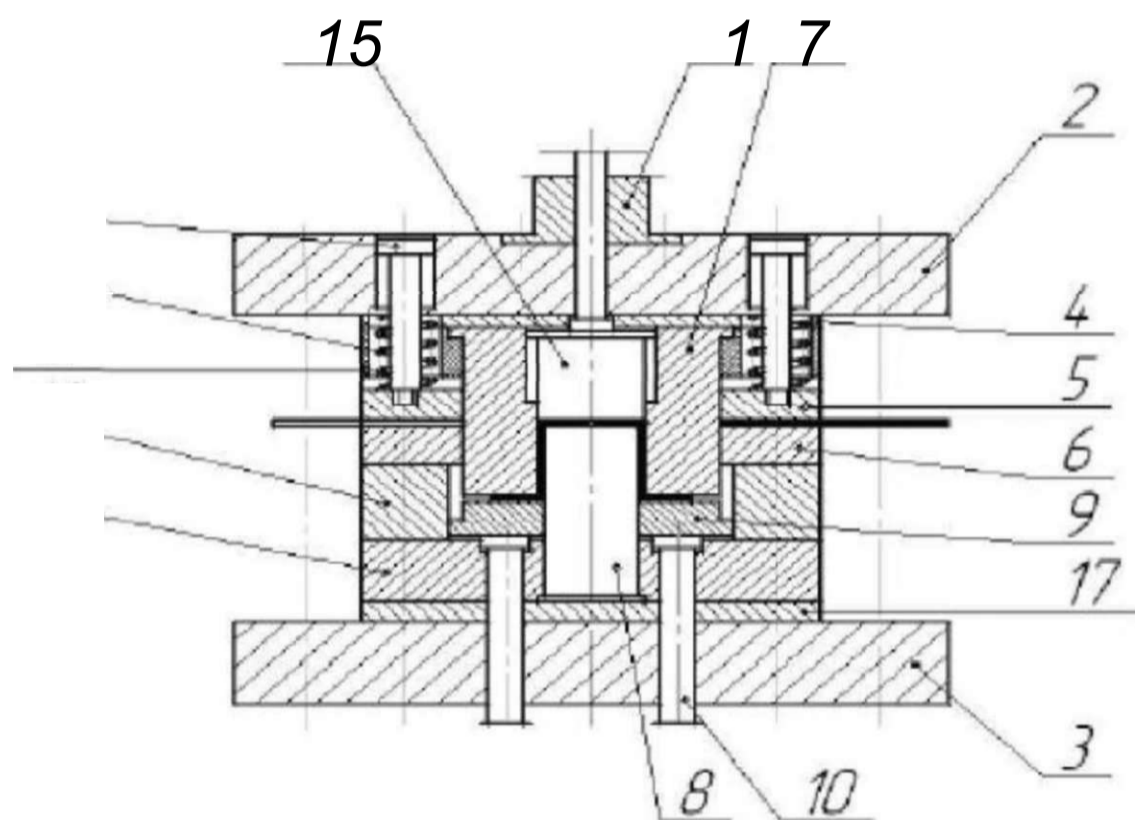
Рис. 5 - Схема штампа совмещённого действия Хля вырубкн и вытяжки
