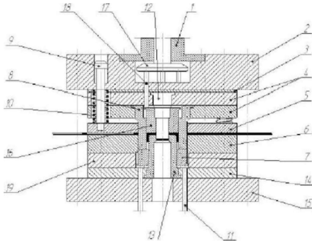
Рис. 1 - Схема штампа совмещенного действия для вырубki, выпллы и пробивки
