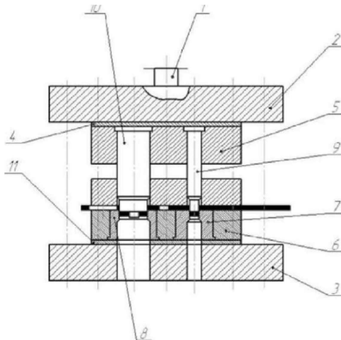
Рис 3-Схема штампа последовательного действия для пробивки и выручки
