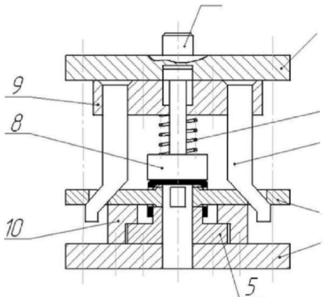
Рис. 11 - Схема клинового штампа для проонвки боковых отверстий
