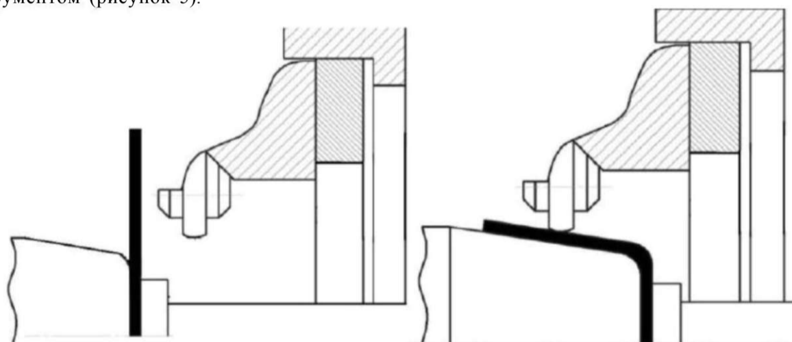
Рисунок 5. Схема раскатки
