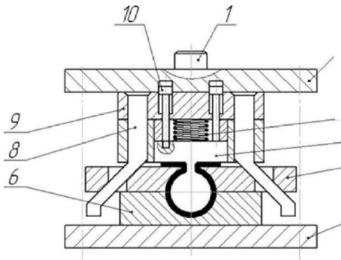
Рис. 10 - Схема клинового штампа для гибки
