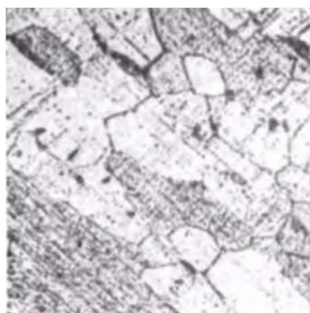
Рис. .93. Микроструктура перегретого дуралюмина. x250.
