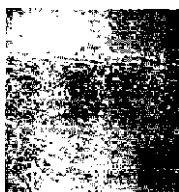
Рис. 5.13. Микроструктура стали (0,65 %С) после лазерной закалки стали. \times 400 .
