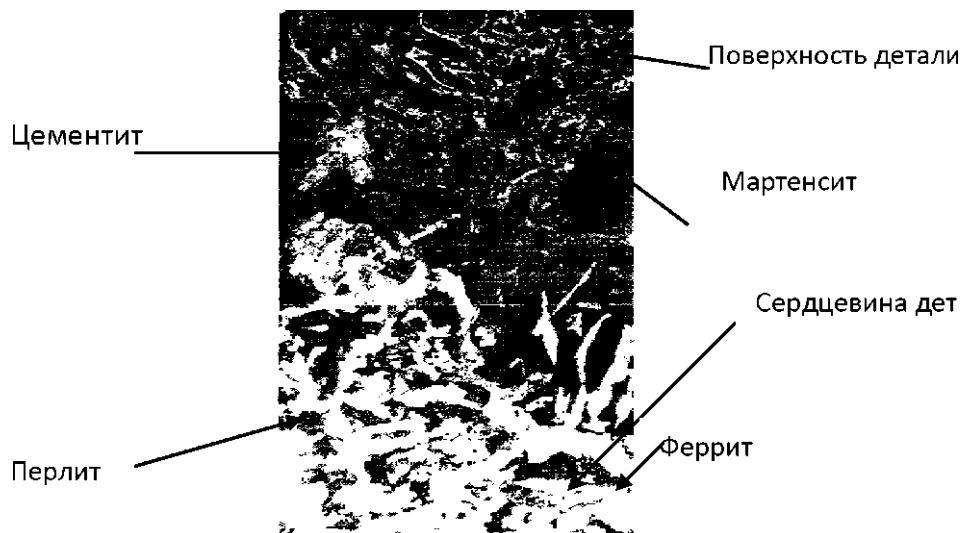
Рис. 5.14. Микроструктура цементованной стали. x200.
