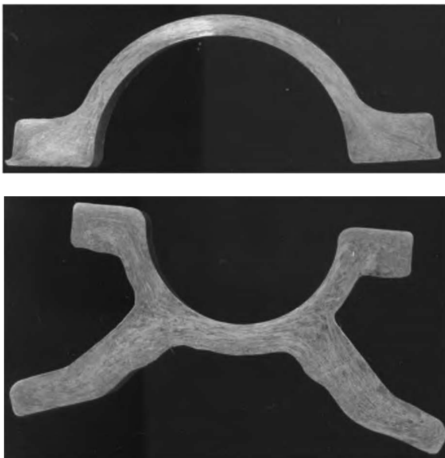
Рис. 12. Макроструктура штампованных поковок. (Верхняя фотография деталь «Крышка», нижняя фотография - деталь «Основание» для сборочного узла «Корпус»).
