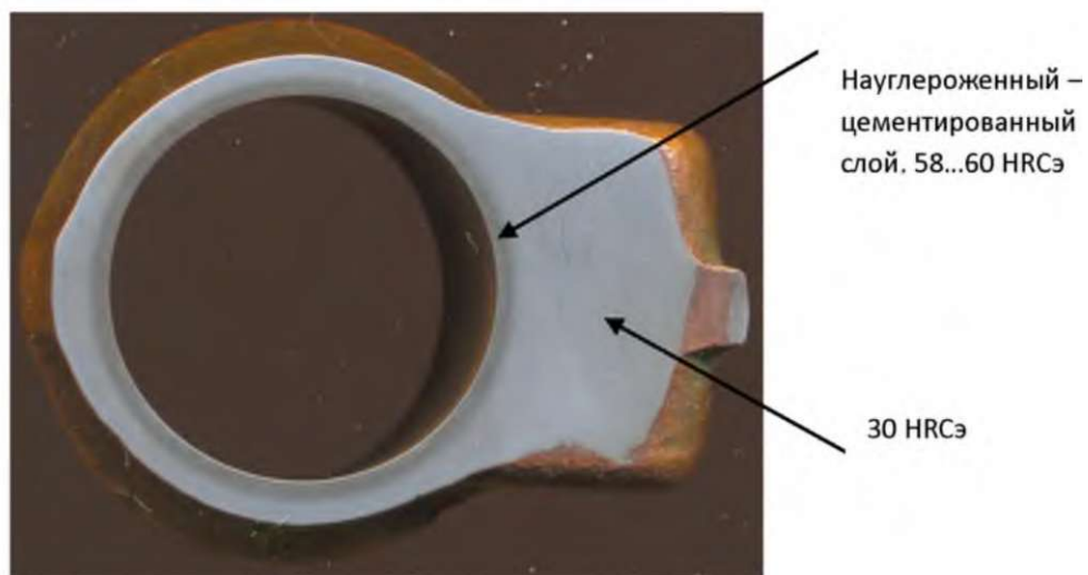
Рис. 8. Макроструктура детали из стали 12ХНЗА с науглероженным (цементированным) слоем.
