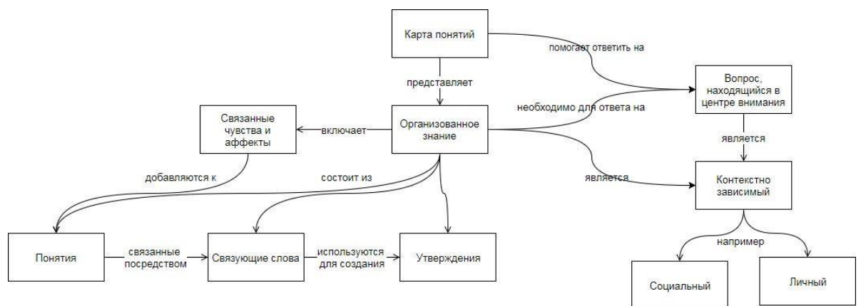
Рис. 7. Карта понятий:
