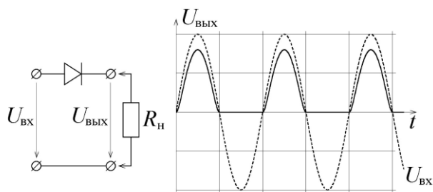
Рис. 2. Однополупериодный выпрямитель и диаграммы его работы
