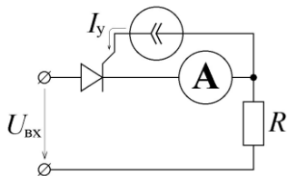
Рис. 7. Измерение напряжения тока тиристора
