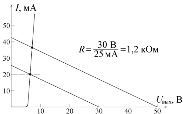
Рис. 3. Проектирование стабилизатора напряжения (пример 1)
