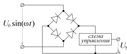
Рис. 8. Измерение параметров выходного сигнала схемы управления
