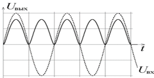
Рис. 4. Диаграммы работы двухполупериодного выпрямителя
