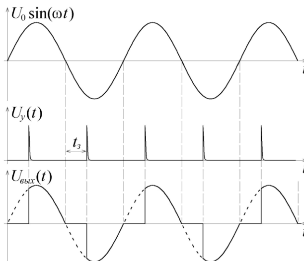
Рис. 6. Диаграммы работы тиристорного регулятора мощности
