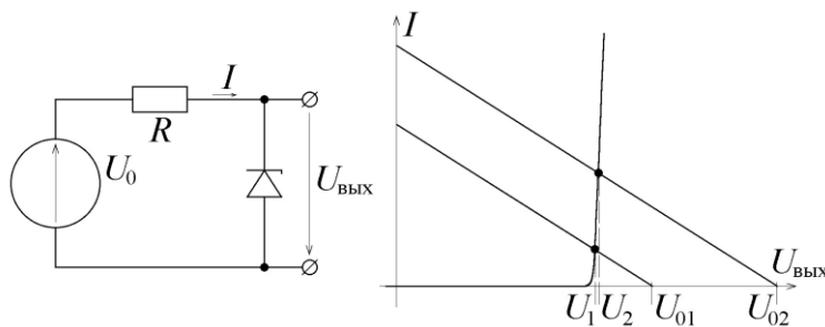
Рис. 2. Параметрический стабилизатор напряжения и принцип его работы
