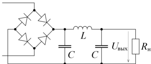
Рис. 7. Индуктивно-емкостной П-образный сглаживающий фильтр
