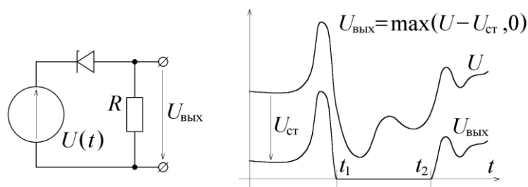
Рис. 14.4. Понижение уровня сигнала на фиксируемую величину
