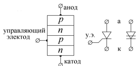
Рис. 1. Структура тиристора и его обозначение
