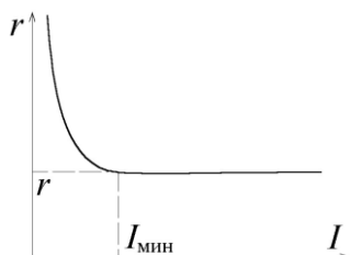
Рис. 14.5. Определение основных параметров стабилитрона
