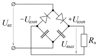
Рис. 8. Удвоитель напряжения Лаггера
