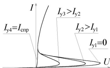
Рис. 2. ВАХ тиристора
