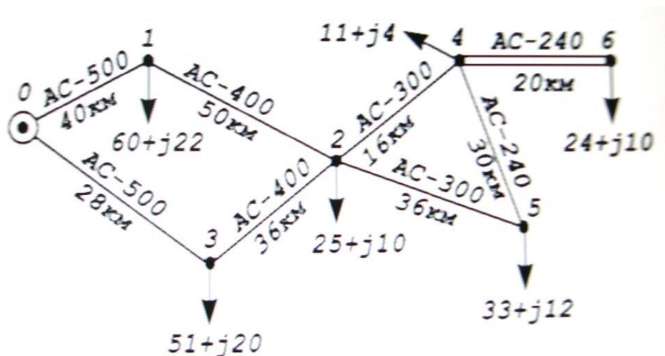
Рис. 5. Схема простой замкнутой кольцевой сети
