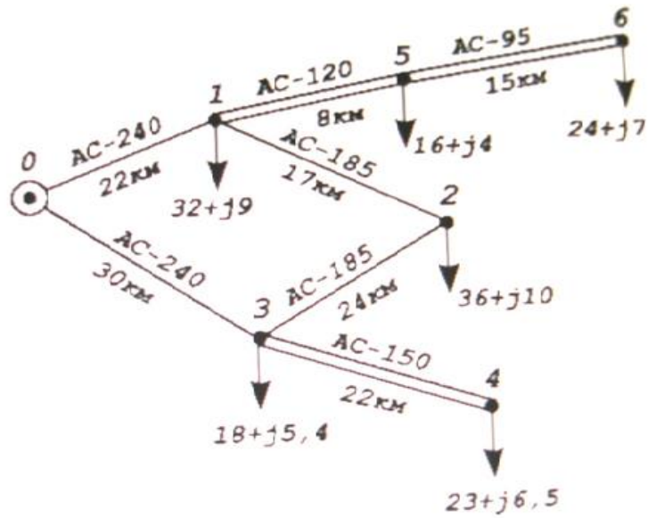
Рис. 1 Схема простой замкнутой кольцевой сети
