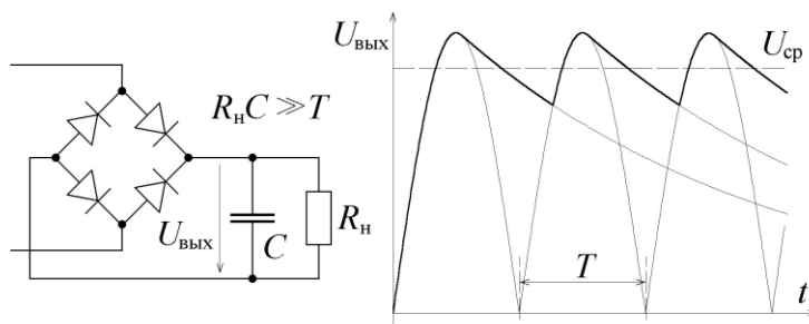
Рис. 5. Емкостной сглаживающий фильтр и диаграммы его работы (без учета падения напряжения на диодах)
