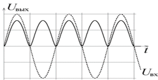
Рис. 4. Диаграммы работы двухполупериодного выпрямителя
