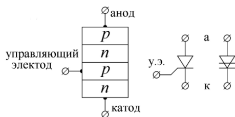
Рис. 1. Структура тиристора и его обозначение
