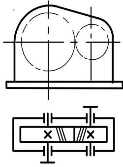
. Схема редуктора.
