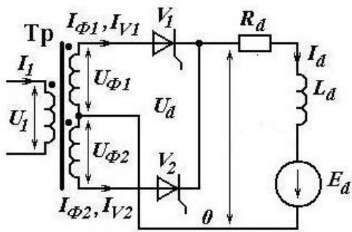
Рис. 1-2 Двухфазная нулевая схема выпрямления
