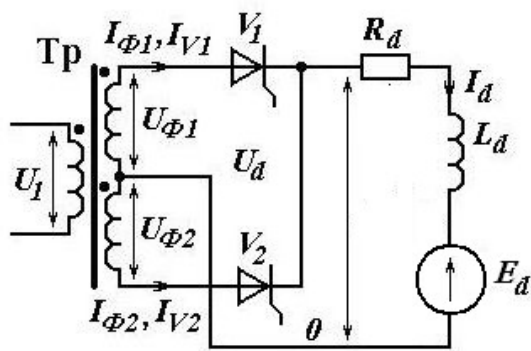
Рис. 1-1 Двухфазная нулевая схема выпрямления
