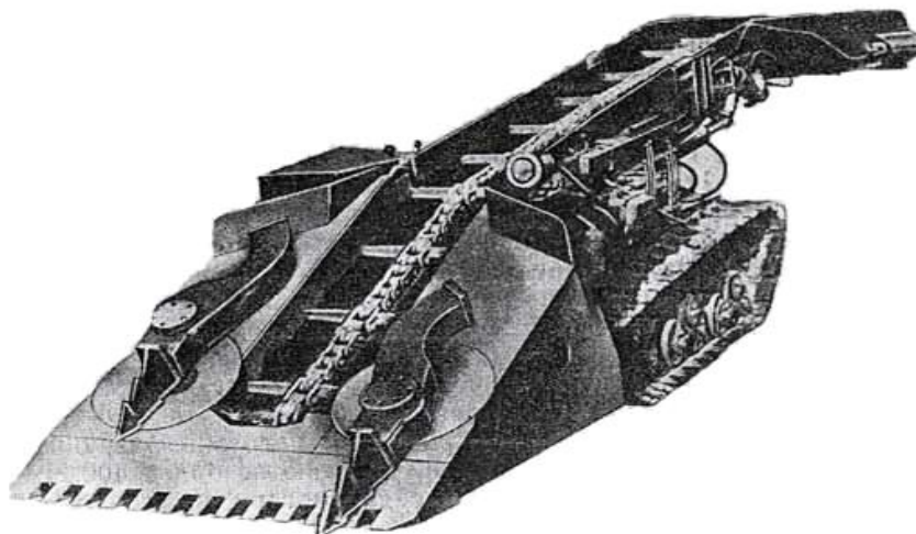
Рис. 29. Погрузочная машина 1ПНБ2
