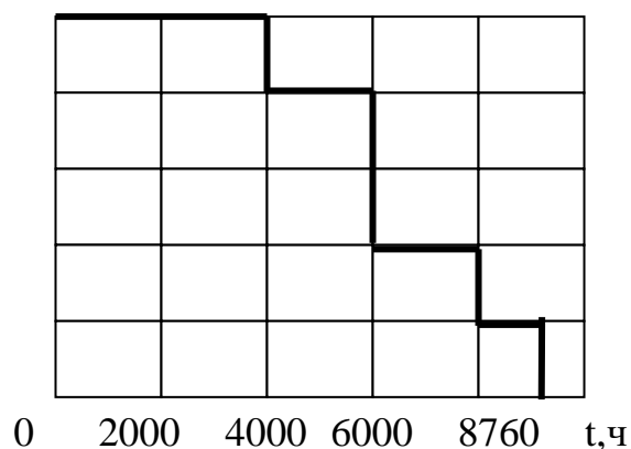
Рис. 1.4. Годовой график нагрузки
