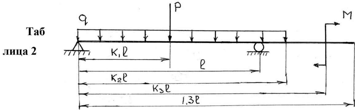
Рис. 0 Типовая схема нагружения балки
