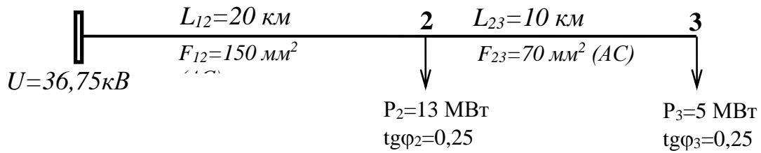
Рис.1. Схема сети
