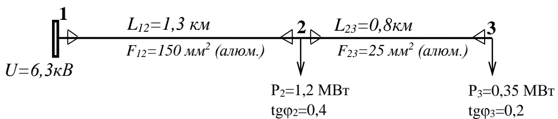
Рис.1. Схема сети
