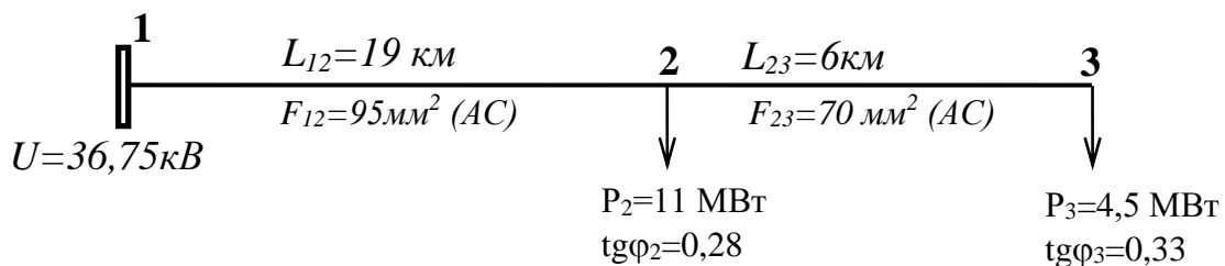
Рис.1. Схема сети
