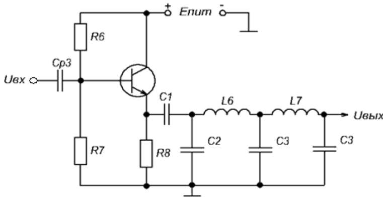
Рис. 17. Принципиальная схема эмиттерного повторителя
