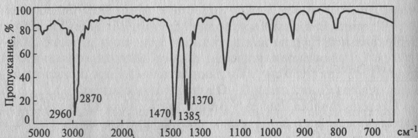
Рис. 5.24. ИК-спектр соединения (жидкая пленка)
