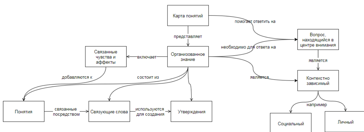
Рис. 7. Карта понятий:
