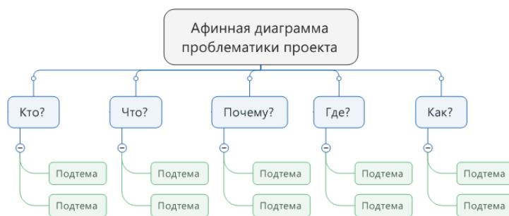
Рис.10. Афинная диаграмма 8 :
