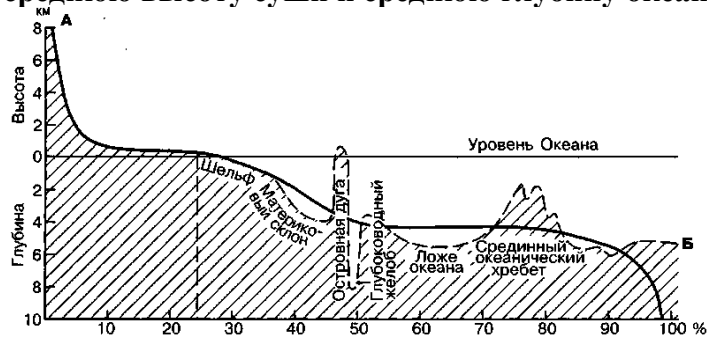
Рисунок 2 – Гипсографическая кривая
