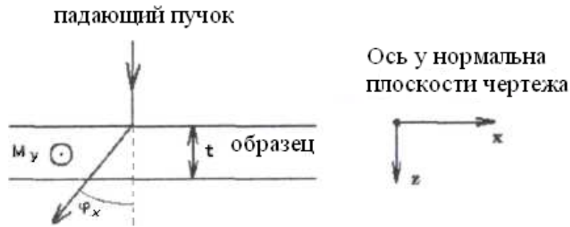
Рис.1.2.1. Отклонение электронного пучка пленкой, намагниченной в направлении y .
