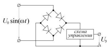
Рис. 8. Измерение параметров выходного сигнала схемы управления
