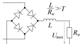
Рис. 6. Индуктивный сглаживающий фильтр.
