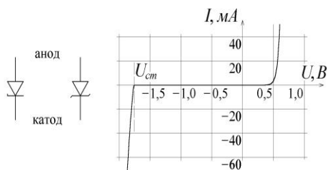
Рис. 1. Условные обозначения стабилитрона (слева — по ГОСТ) и типичный вид его вольт-амперной характеристики
