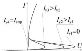
Рис. 2. ВАХ тиристора
