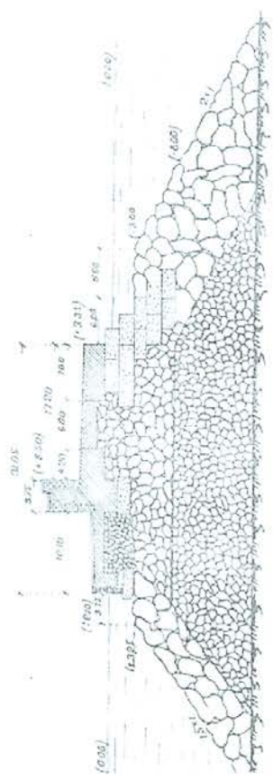
Рис.20 Генуэзский порт, Миловой профиля мола Дуллиера
