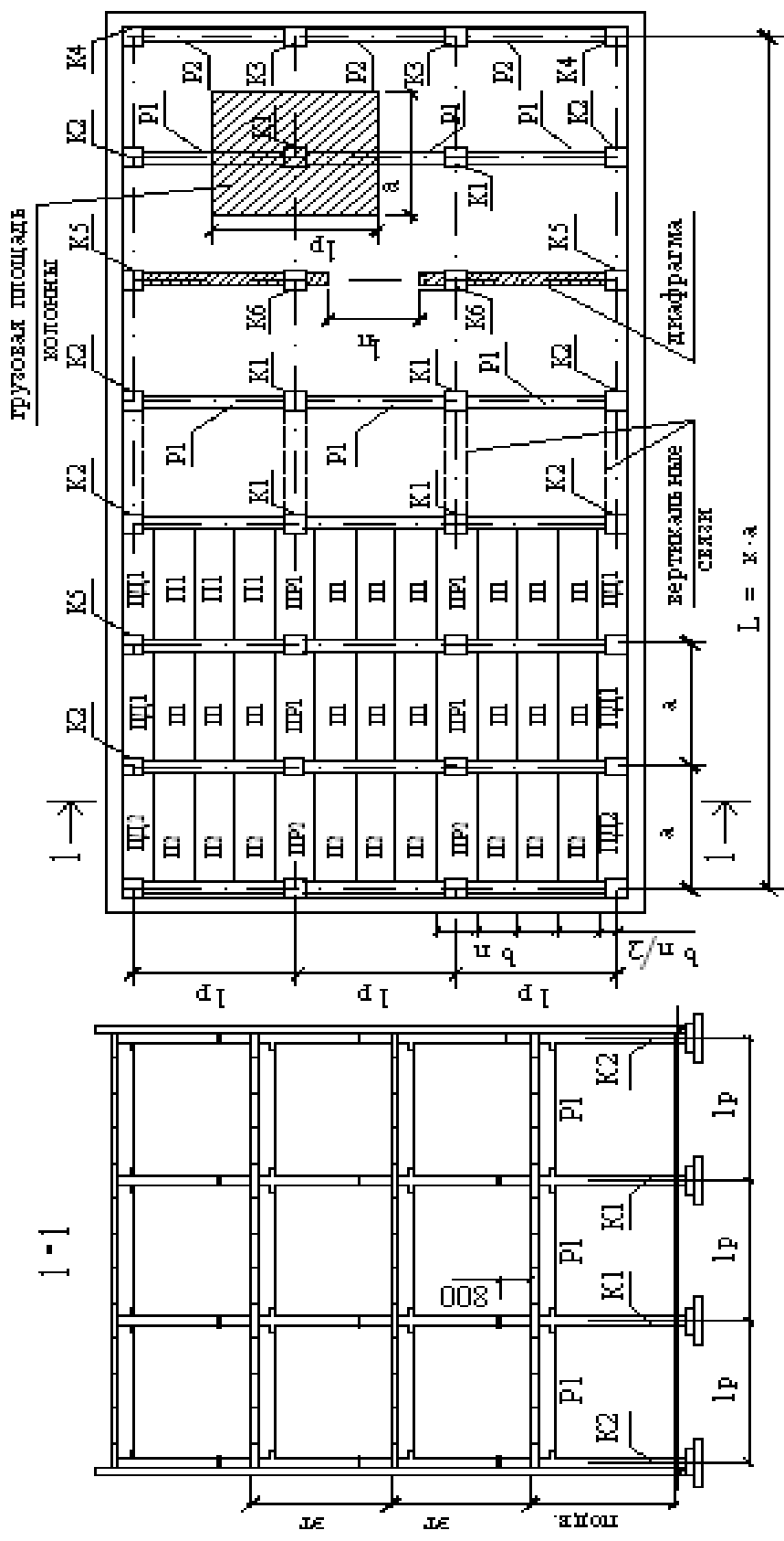
Рисунок 1. Конструктивный разрез и совмещенный план перекрытия
