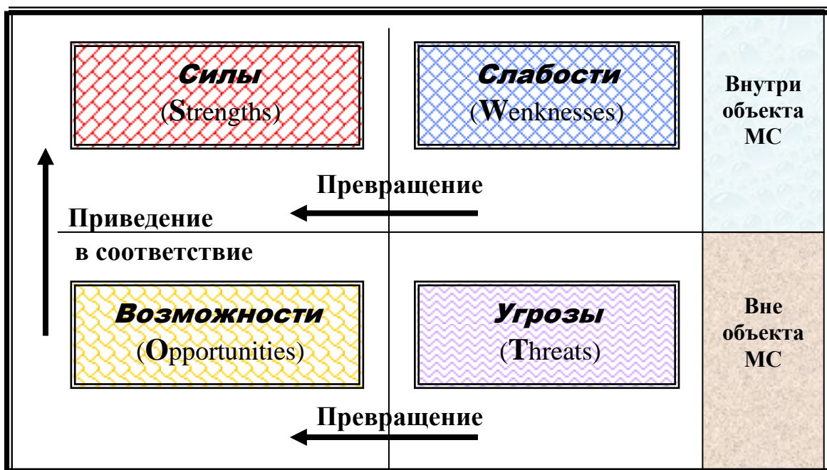
Рисунок 2 - Схема SWOT-анализа
