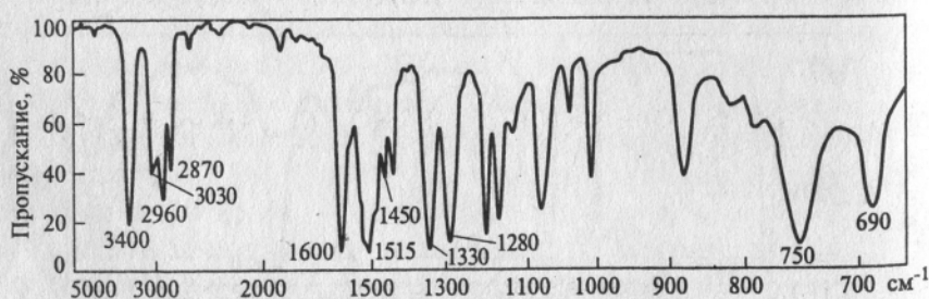
Рис. 5.22. ИК-спектр N -метиланилина (жидкая пленка)
