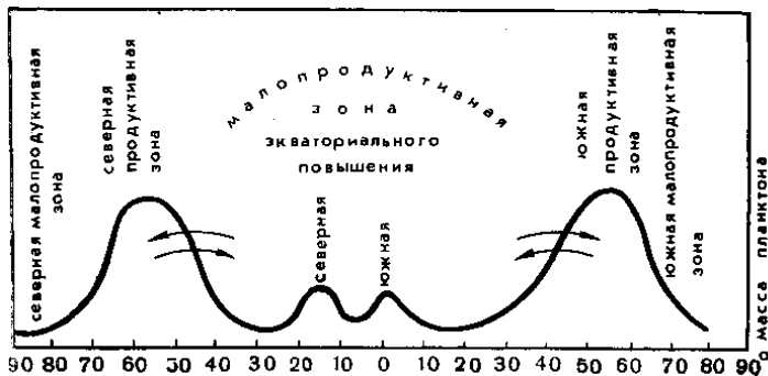
Рисунок 8 – Схема биологической продуктивности Мирового океана.
