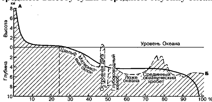
Рисунок 2 – Гипсографическая кривая
