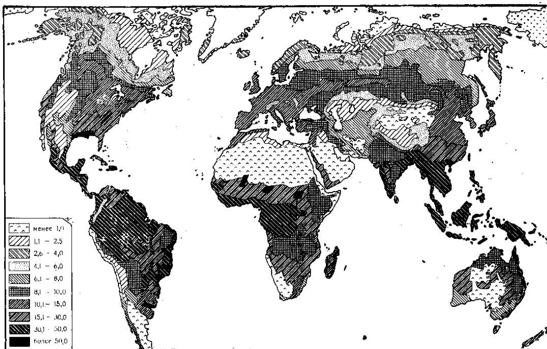
Рисунок 7 – Ежегодный прирост органического вещества растительности на земной поверхности, t/га
