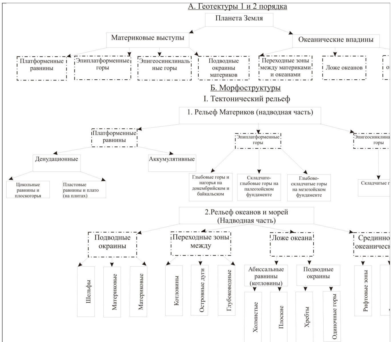
Рисунок 6 – Генетическая классификация форм эндогенного рельефа (по Любушкиной С.Г.)
