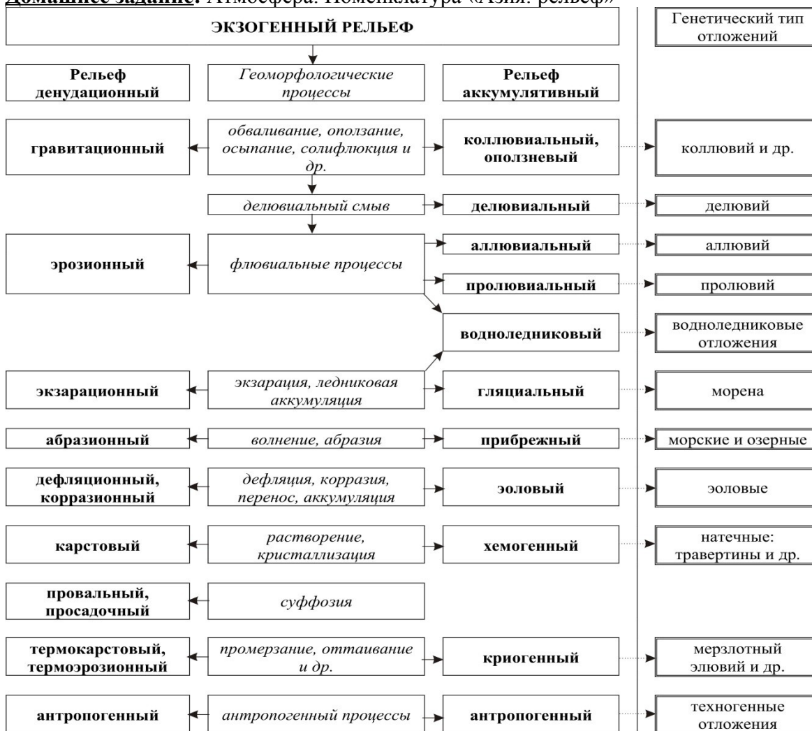
Рисунок 5 – Генетическая классификация типов экзогенного рельефа (по Любушкиной С.Г.)
