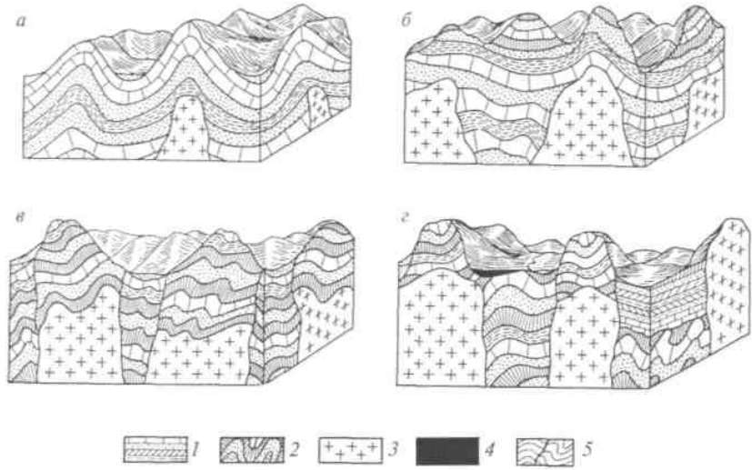
Рисунок 3 – Типы (А – Д) морфоструктур равнинных областей (по Пашкангу К.В.)
