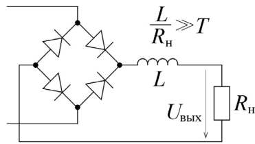
Рис. 6. Индуктивный сглаживающий фильтр.
