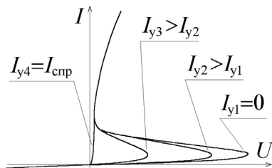
Рис. 2. ВАХ тиристора
