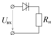
Рис. 2. Тиристор снагрузкой
