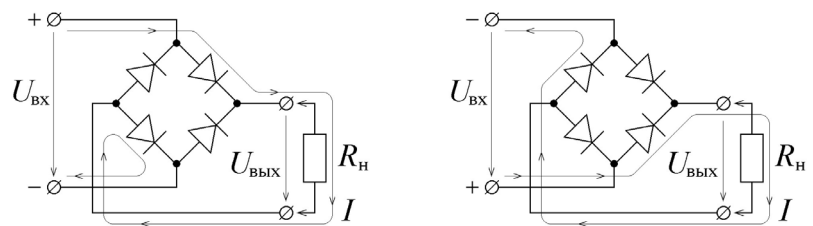
Рис. 3. Двухполупериодный выпрямитель. Показан путь протекания электрического тока при различных полярностях входного напряжения
