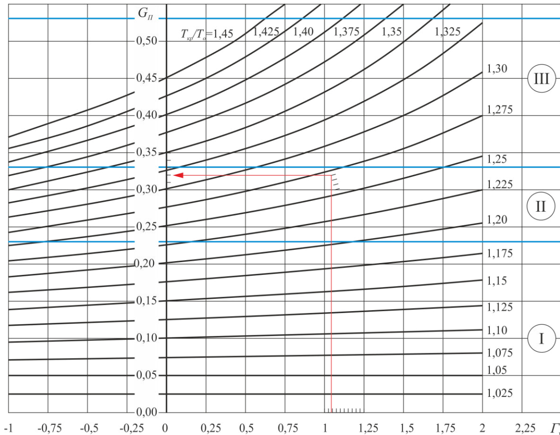
Рис. 3. Номограмма для определения группы пожароопасности скопления угля пласта l_1 для G_v = 1,043 и T_{sp}/T_o = 1,27 .
