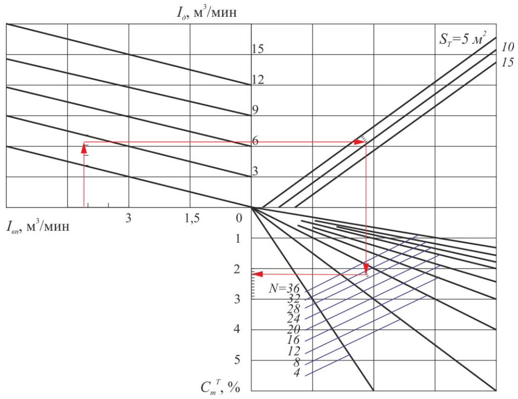
Рис. 3. Номограмма для определения C_m^T .
