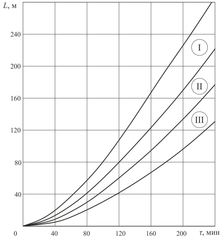
Рис. 2. Дальность распространения подземных пожаров в зависимости от их класса (I, II, III).
