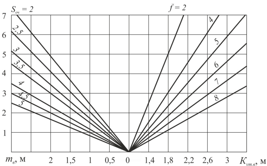
Рис. 1. Номограмма для определения k_{ум.в}
