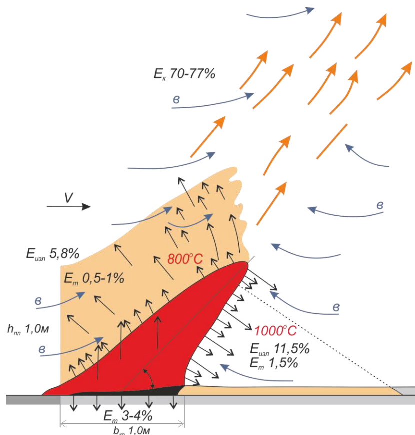
Рис. 4.1. Схема рассеивания тепла горящей кромкой низового пожара: E_k , E_{изл} , E_m – потери тепла конвекцией, излучением, теплопроводностью.
