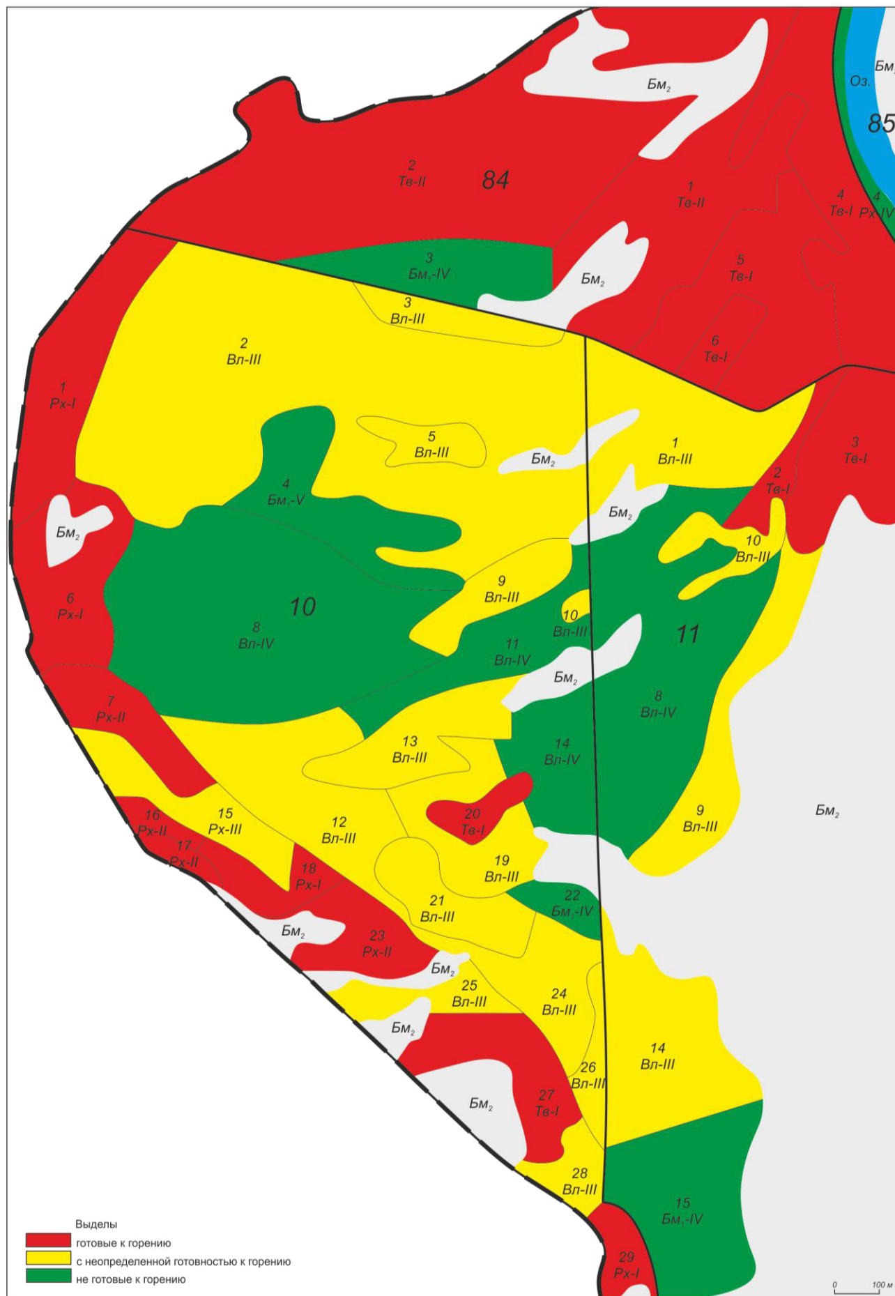
Рис. 2.3. Карта «пожарной зрелости» при III классе засухи.
