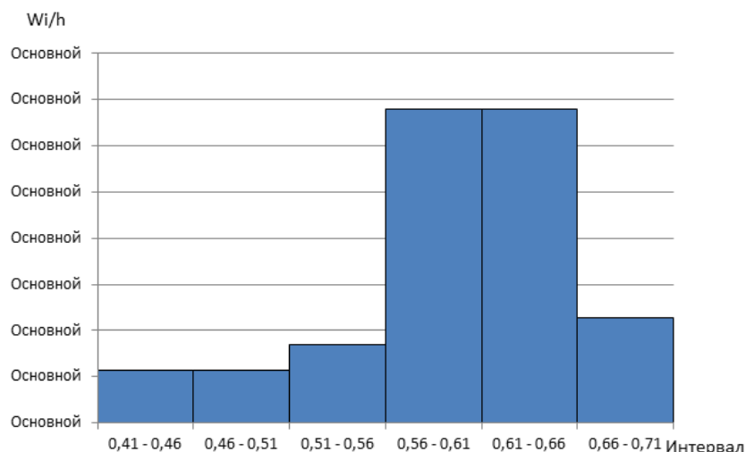
Рисунок 3 – Гистограмма частот
