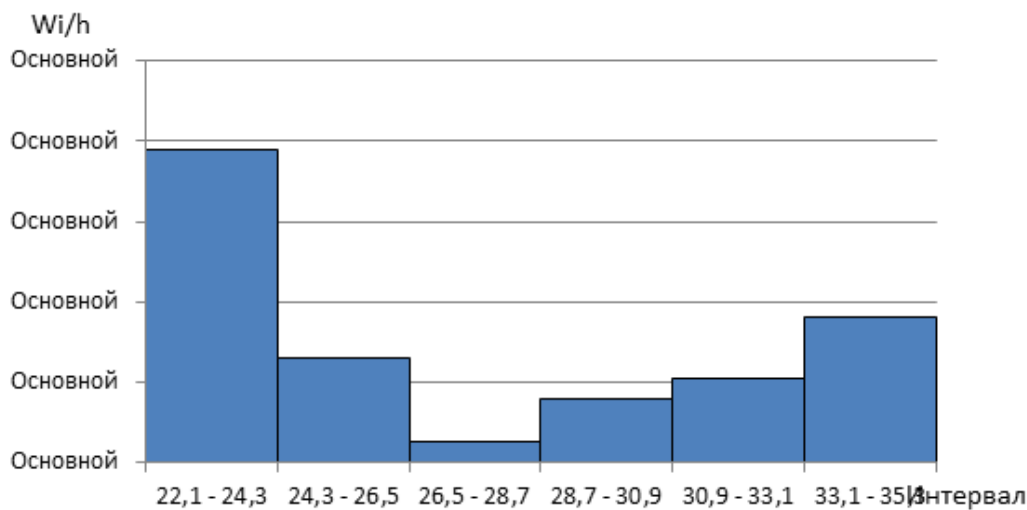
Рисунок 2 – Гистограмма частот
