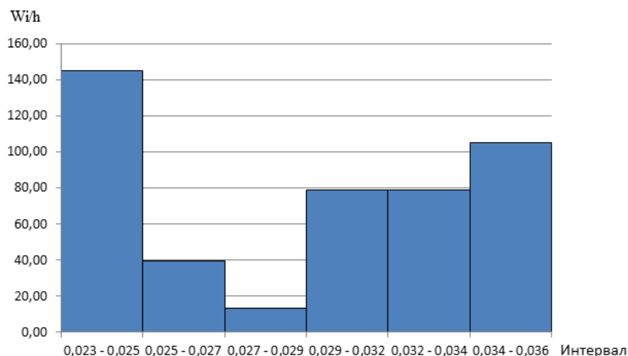
Рисунок 4 – Гистограмма частот
