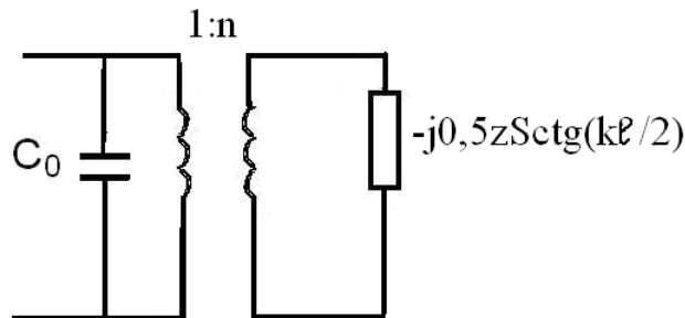
Рис. 2 Эквивалентная схема стержневого преобразователя без учета потерь
