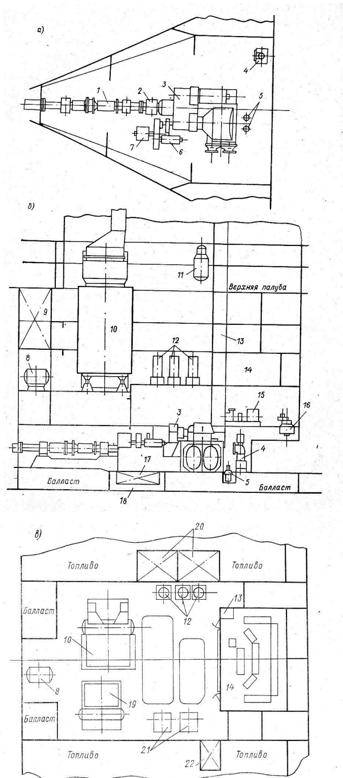
Схема расположения основного оборудования ПТУ танкеров типа «Крым»: а — план трюма; б — продольный разрез, вид на левый борт; в — план платформы
