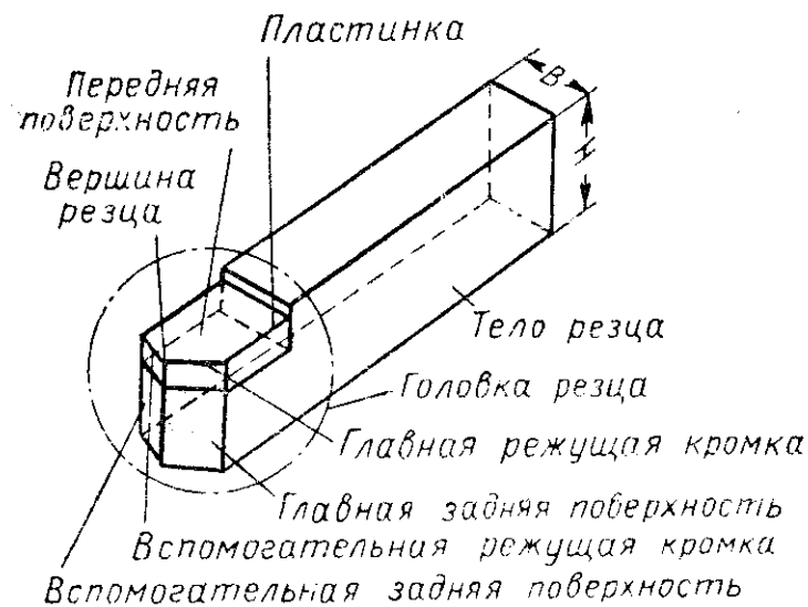
Рис. 1. Элементы резца
