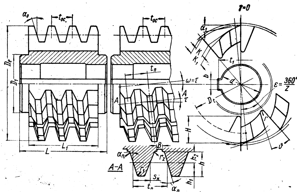
Рис. 36. Конструктивные элементы червячных фрез
