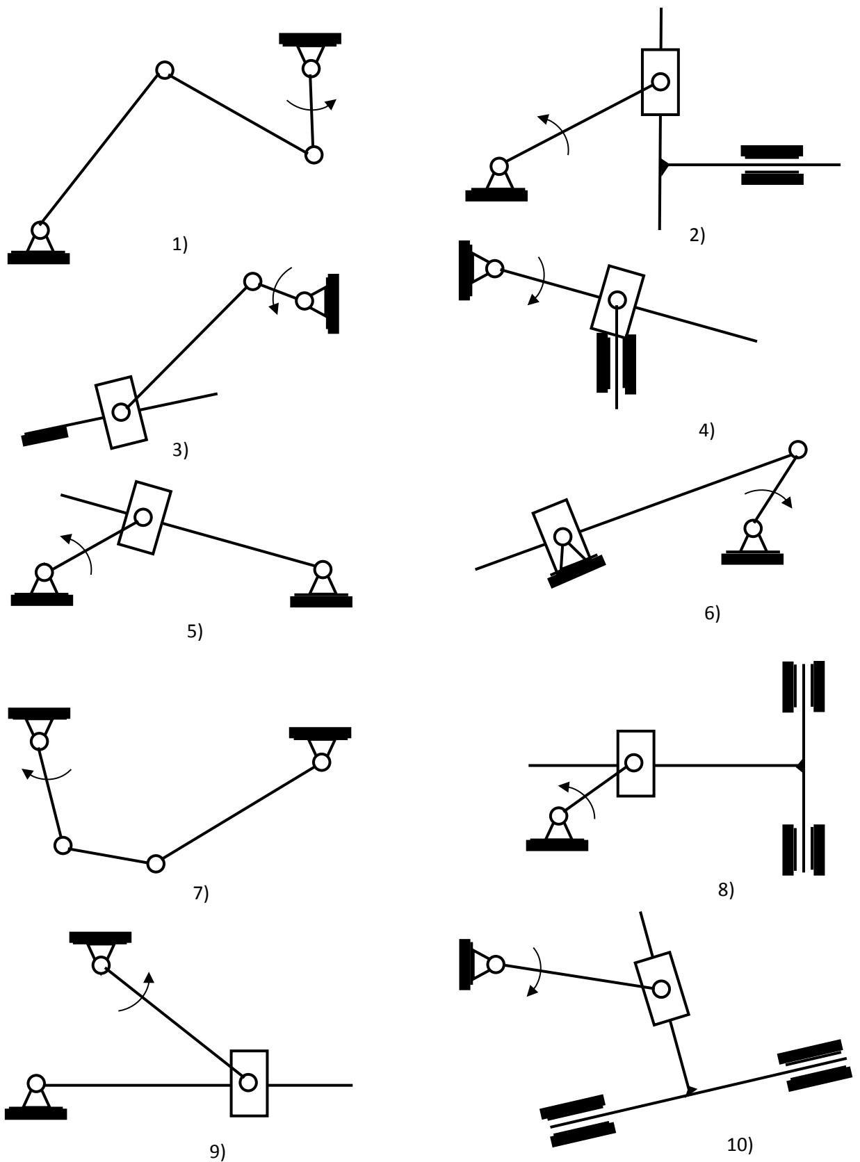
Рис. 1 Схемы четырехзвенных плоских механизмов
