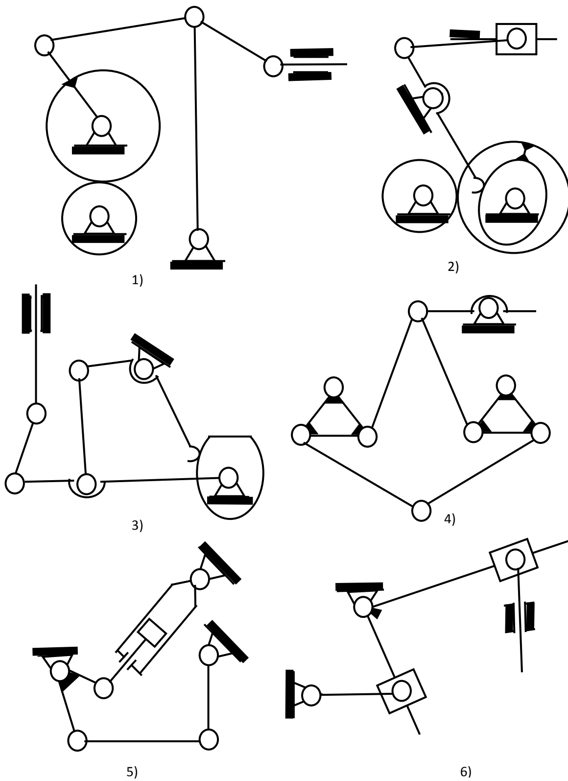
Рис. 1.6. Кинематические схемы плоских механизмов
