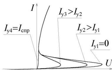
Рис. 2. ВАХ тиристора
