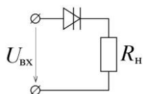
Рис. 2. Тиристор снагрузкой
