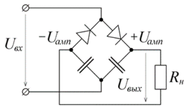
Рис. 8. Удвоитель напряжения Лаггера
