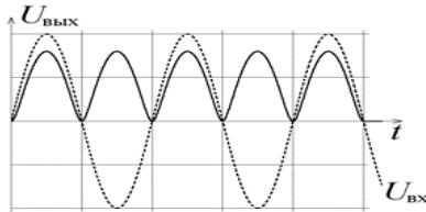
Рис. 4. Диаграммы работы двухполупериодного выпрямителя
