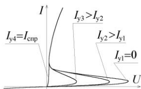
Рис. 2. ВАХ тиристора
