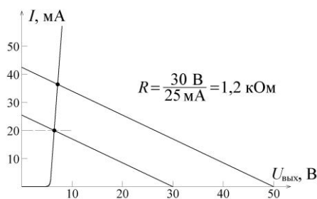
Рис. 3. Проектирование стабилизатора напряжения (пример 1)
