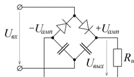
Рис. 8. Удвоитель напряжения Лаггера
