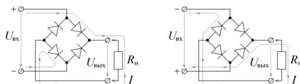
Рис. 3. Двухполупериодный выпрямитель. Показан путь протекания электрического тока при различных полярностях входного напряжения
