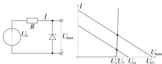
Рис. 2. Параметрический стабилизатор напряжения и принцип его работы
