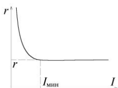
Рис. 14.5. Определение основных параметров стабилитрона
