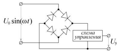
Рис. 8. Измерение параметров выходного сигнала схемы управления
