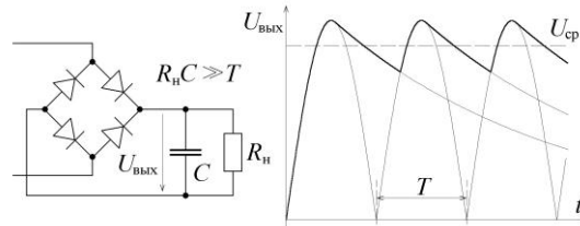
Рис. 5. Емкостной сглаживающий фильтр и диаграммы его работы (без учета падения напряжения на диодах)
