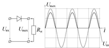
Рис. 2. Однополупериодный выпрямитель и диаграммы его работы
