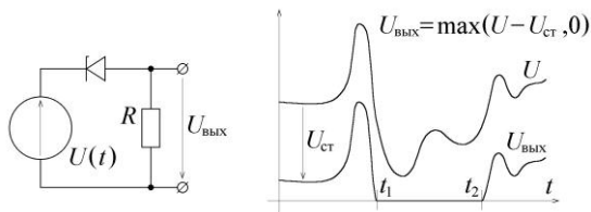
Рис. 14.4. Понижение уровня сигнала на фиксируемую величину
