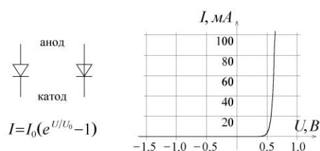
Рис. 1. Обозначения полупроводникового диода и типичный вид его вольт-амперной характеристики
