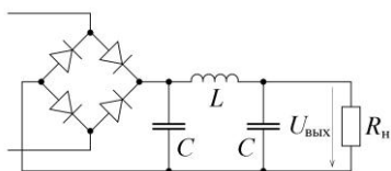
Рис. 7. Индуктивно-емкостной П-образный сглаживающий фильтр
