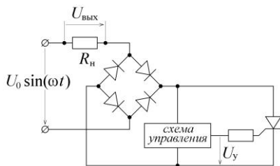
Рис. 5. Тиристорный регулятор мощности
