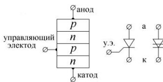
Рис. 1. Структура тиристора и его обозначение
