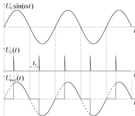
Рис. 6. Диаграммы работы тиристорного регулятора мощности
