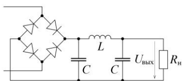
Рис. 7. Индуктивно-емкостной П-образный сглаживающий фильтр
