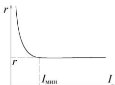
Рис. 14.5. Определение основных параметров стабилитрона
