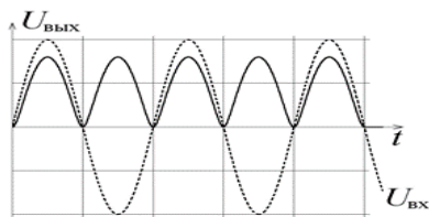
Рис. 4. Диаграммы работы двухполупериодного выпрямителя
