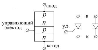
Рис. 1. Структура тиристора и его обозначение
