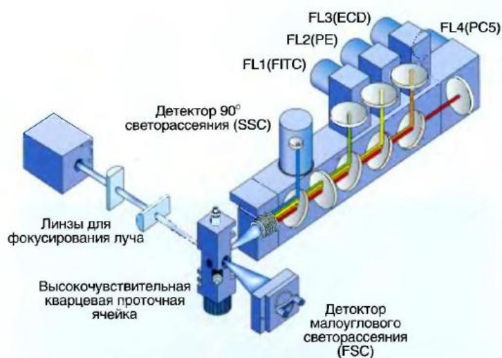
Рис. 2.4. Устройство проточного цитометра
